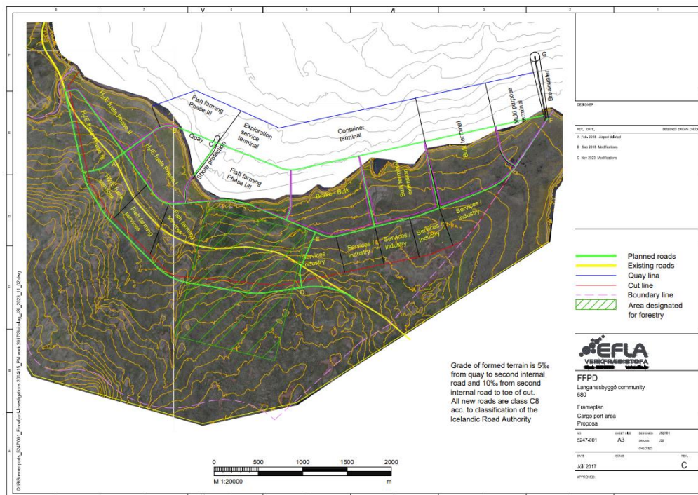
Rammaskipulag fyrir Farnafjarðarhöfn (frumdrög).
